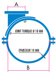
Collier départ tangentiel Nous consulter
