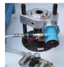
Motorisation pneumatique
