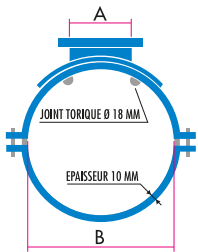
Collier bride fixe
