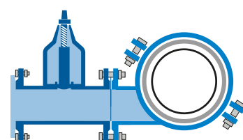
Percement tangentiel (Piquage bas, au fil de l'eau)
