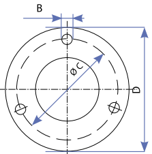
Un trou doit toujours se trouver sur l'axe vertical et à la partie supérieure de la bride
