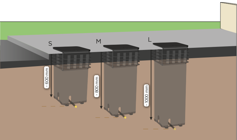
Résistance au gel testée par le Laboratoire CEREMA
