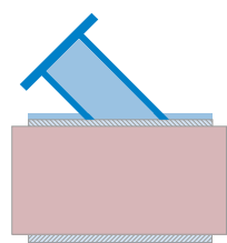
Percement à 45° (Introduction d'une sonde ou sortie à 45°) Autres angles : nous consulter
