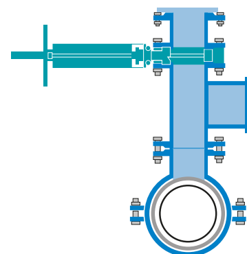
Percement par le dessus (Réseaux encombrés)
