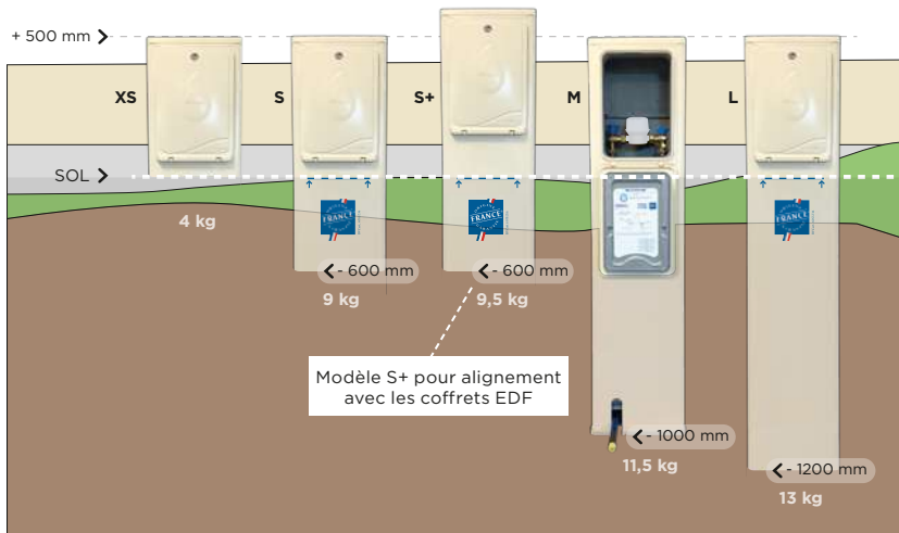
Hauteur d'enfouissement en fonction de la zone de gel
