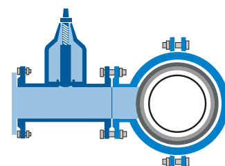
Percement sur tuyau Bonna (Cas d'un tuyau à âme tôle : étanchéité sur l'âme tôle)
