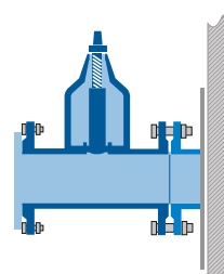
Percement en applique (Percement d'une conduite ovoïde ou sur un réservoir)
