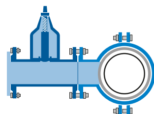
Percement horizontal (Configuration classique)
